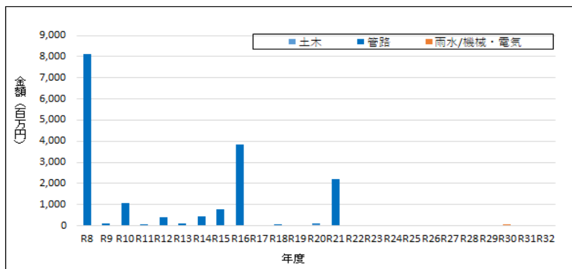
図 4-12 将来の雨水施設更新需要(法定耐用年数で更新)
