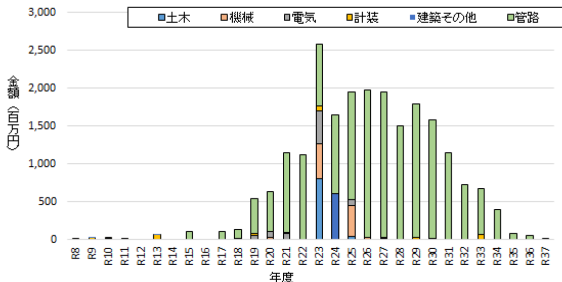
図 4-11 将来の污水施設更新需要(法定耐用年数で更新)
