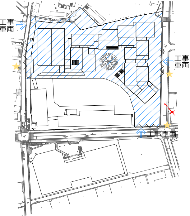
【STEP2】校舎・体育館棟建設工事中 (令和8年10月～令和10年2月末)
