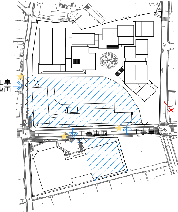
【STEP3】校舎と既存体育館解体改修工事中 (令和10年5月～9月末)
