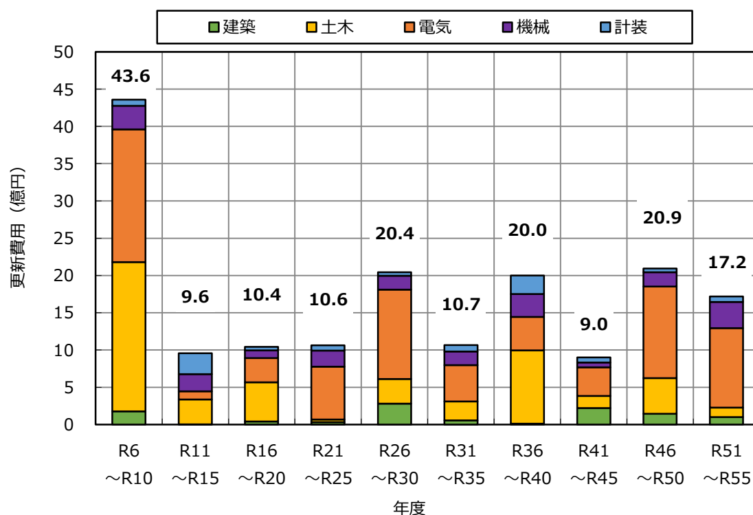
図 3-5 浄配水場・設備の更新費用
