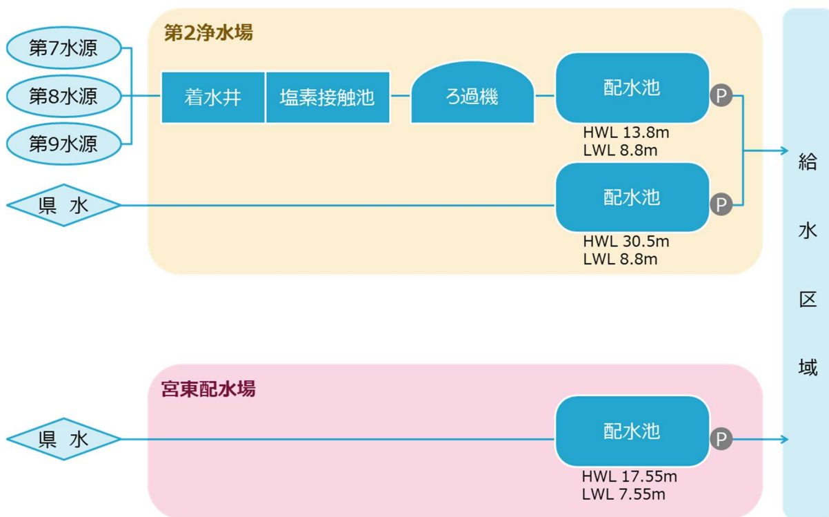
図 2-2 配水系統図
