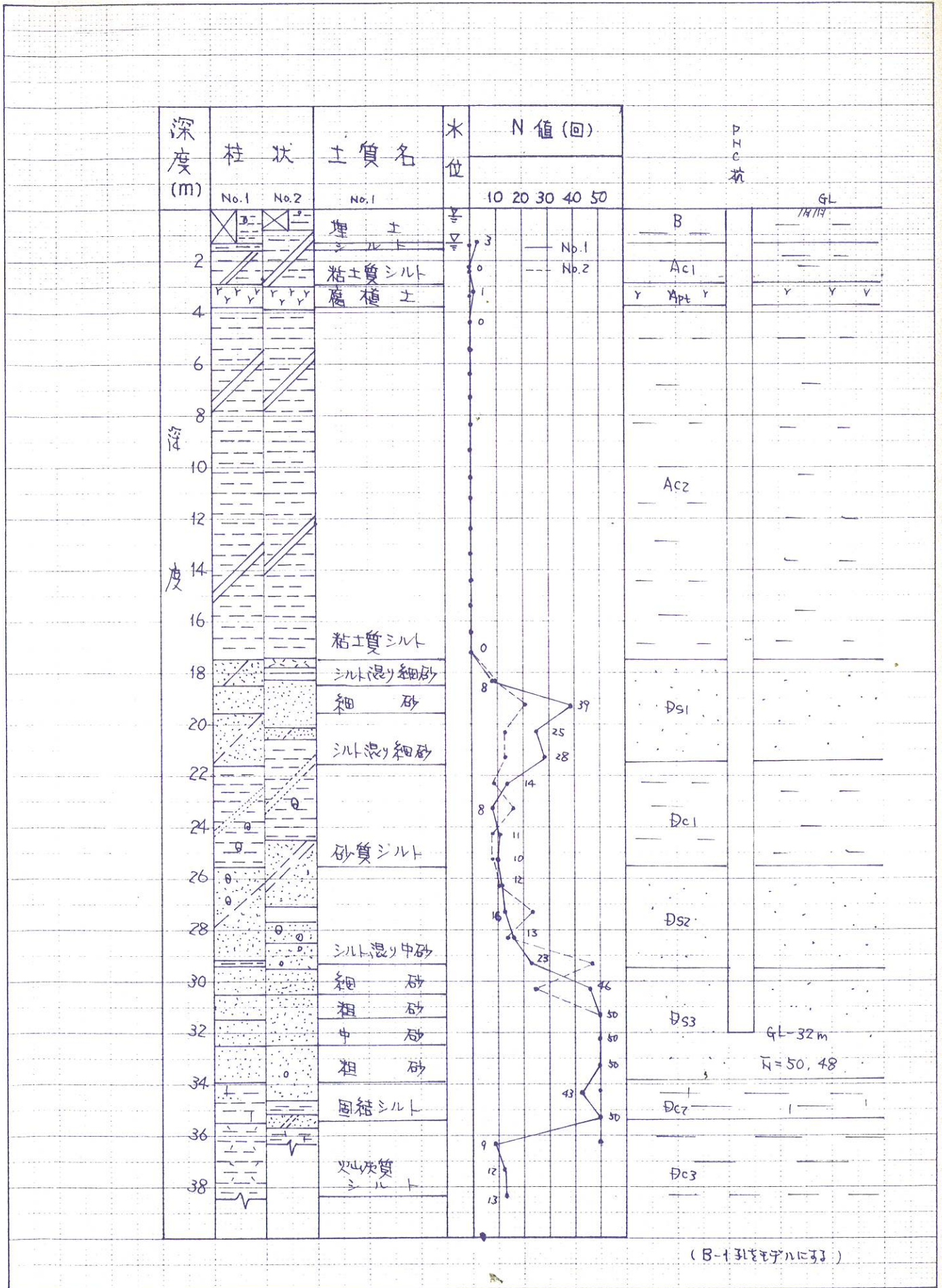
図4-1 杭の打設深度図
