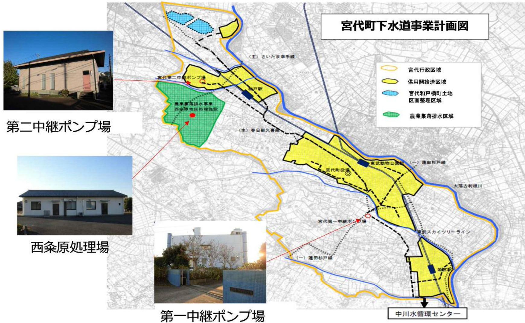
図3-1 施設概要図
