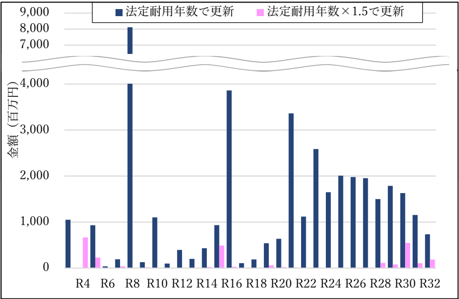
耐用年数の設定による更新需要比較（公共下水道） P31 参照
