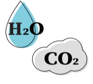
水とCO 2 に分解
