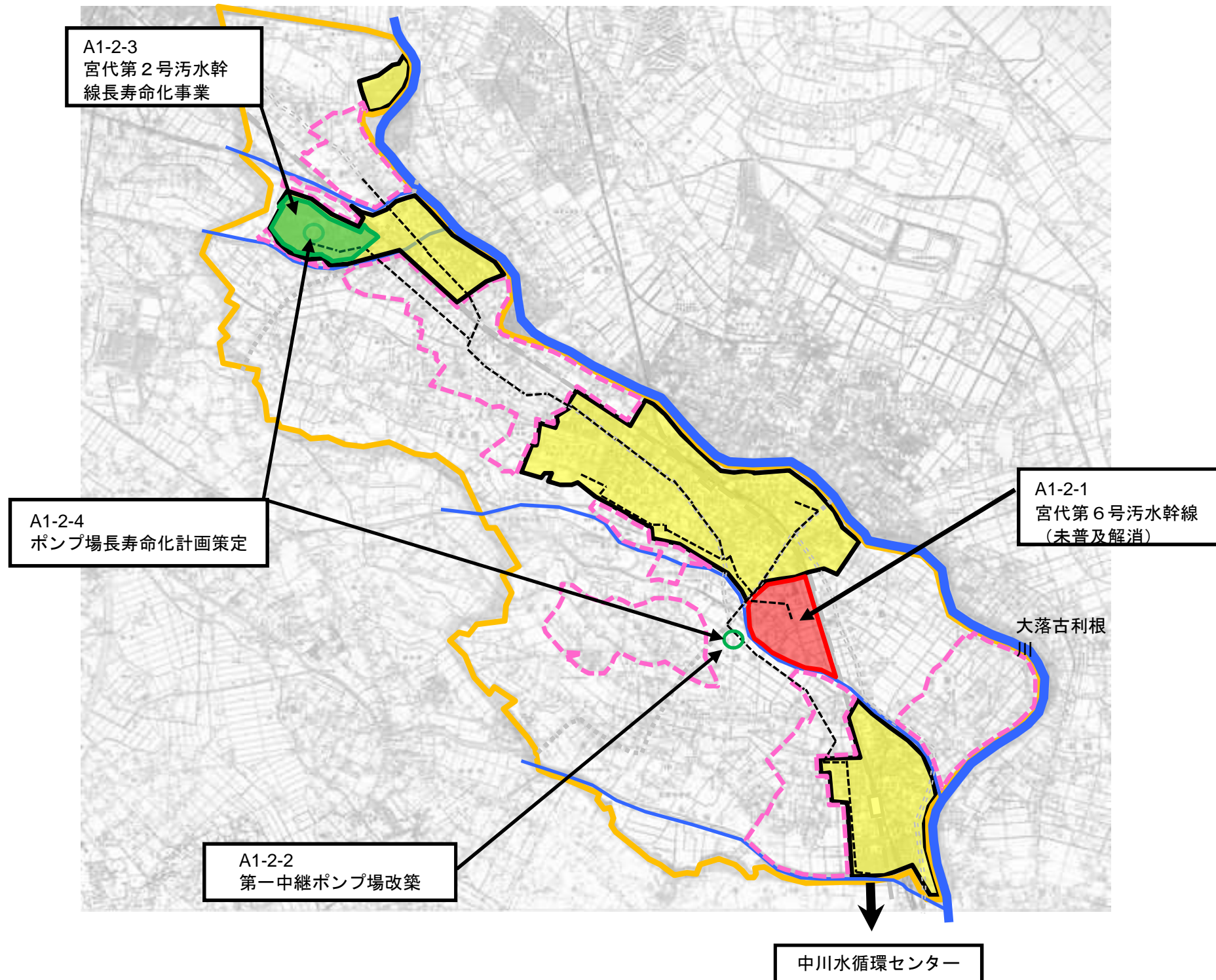
中川処理区計画図
