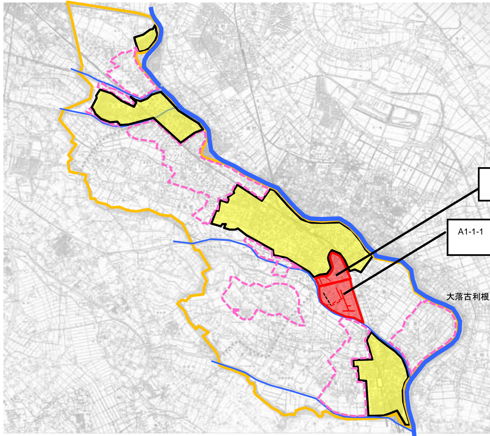
中央排水区計画図
